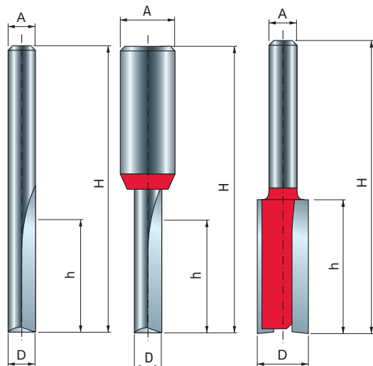
Typ A Frezy monolityczne
