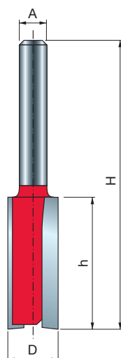
Typ C Frezy z ostrzami węglikowymi
