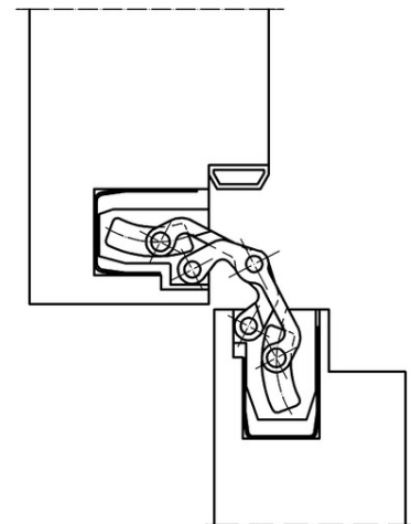
ościeżnica blokowa drewniana 90°
