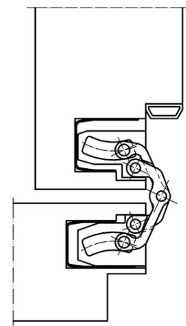
ościeżnica blokowa drewniana 180°
