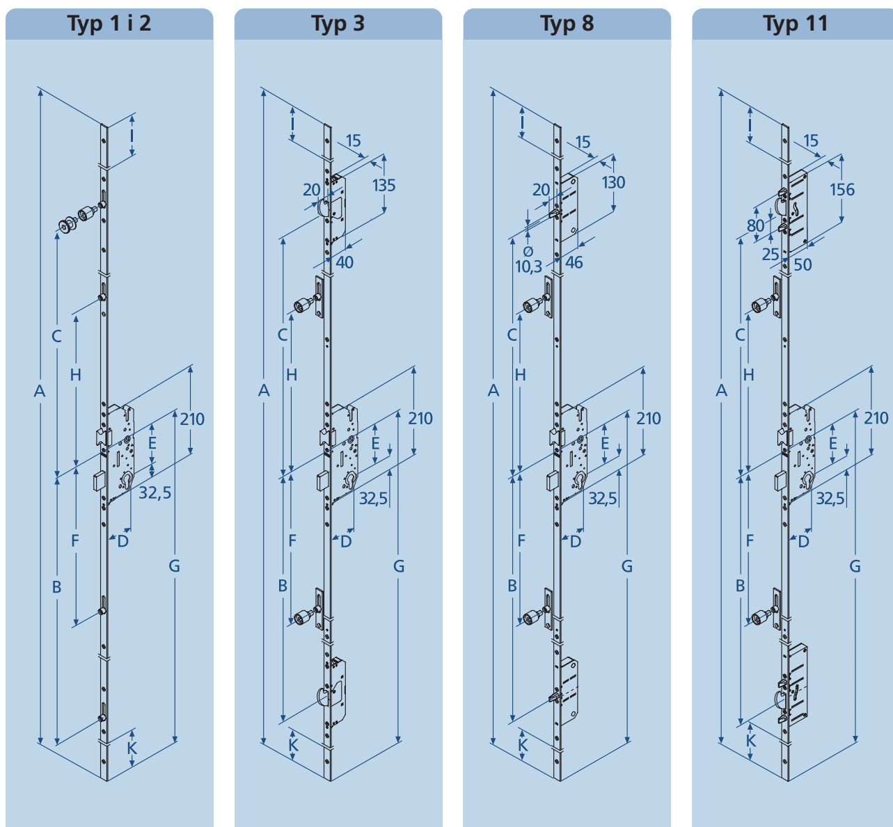
Wymiary Typ 1 i 2
